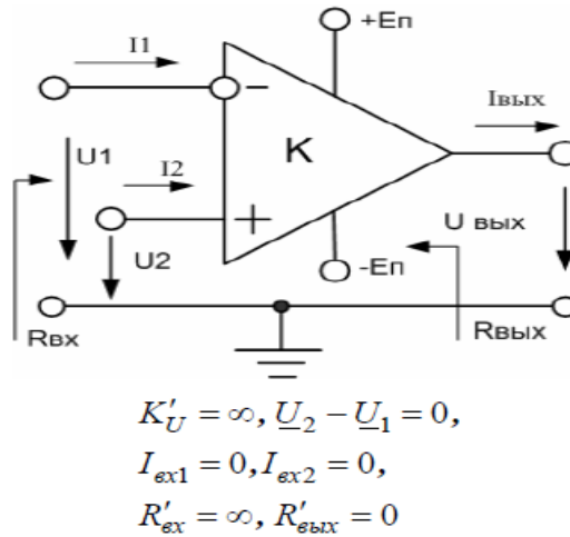
Рисунок 2. Идеальный ОУ
