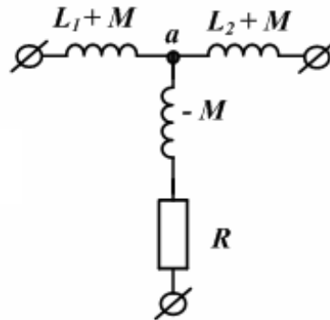
Рисунок 6. Эквивалентная схема с тремя индуктивностями без магнитной связи
